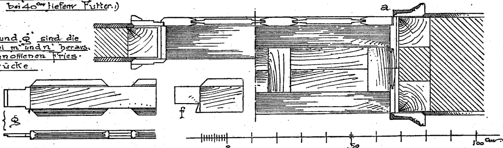
Gestemmte einflügelige Zimmerthüre.
